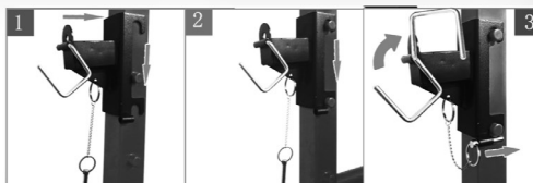
Způsob montáže držáku na činku.
